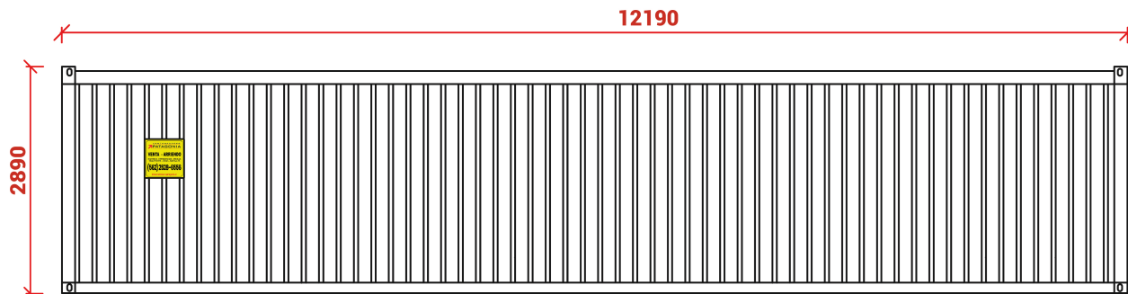
Elevación Sur
