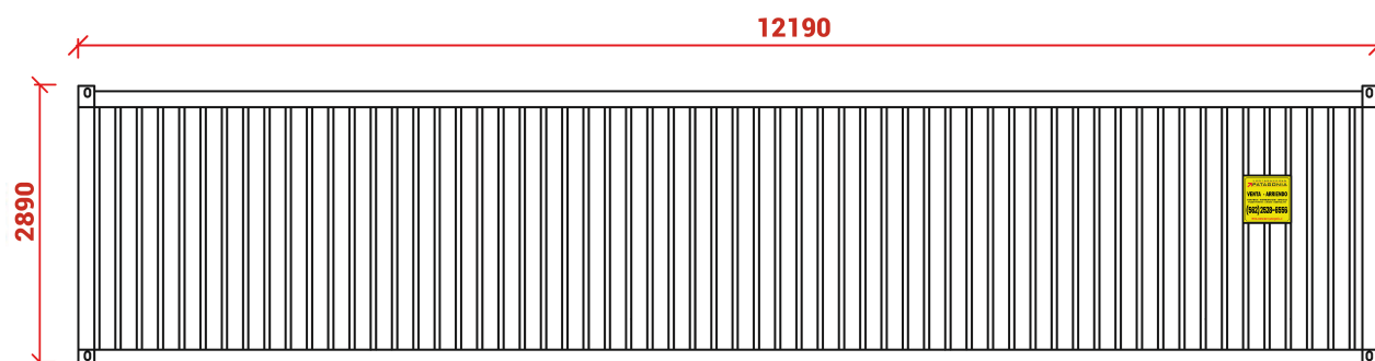
Elevación Norte
