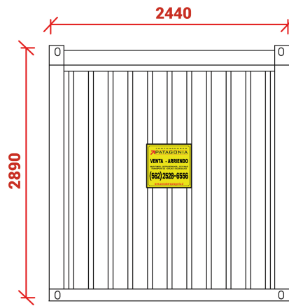
Elevación Oeste
