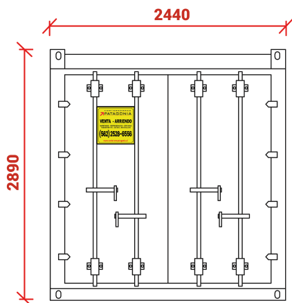
Elevación Este
